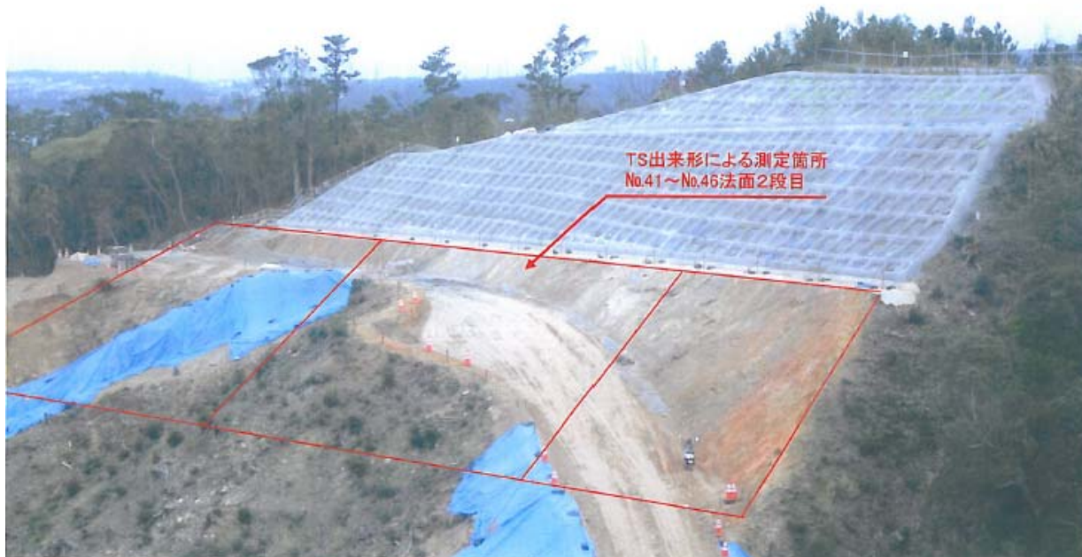
TSによる出来形管理デモンストレーション
